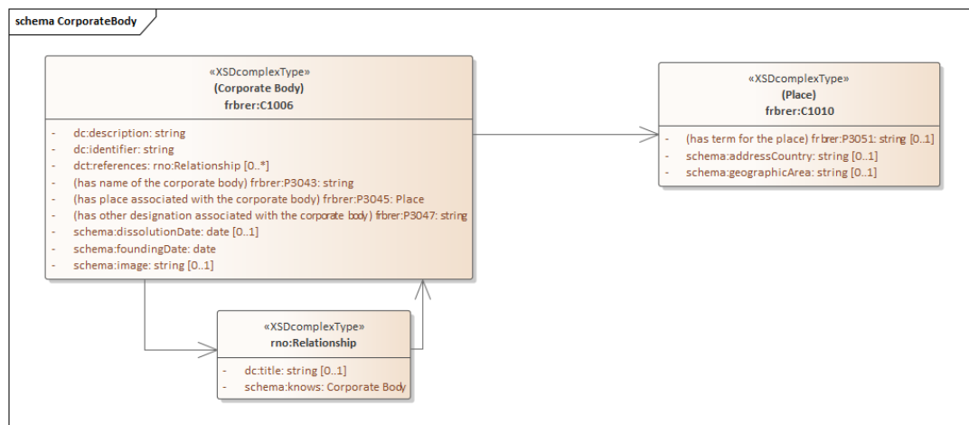
Figura 4 Ontología Corporate Body
