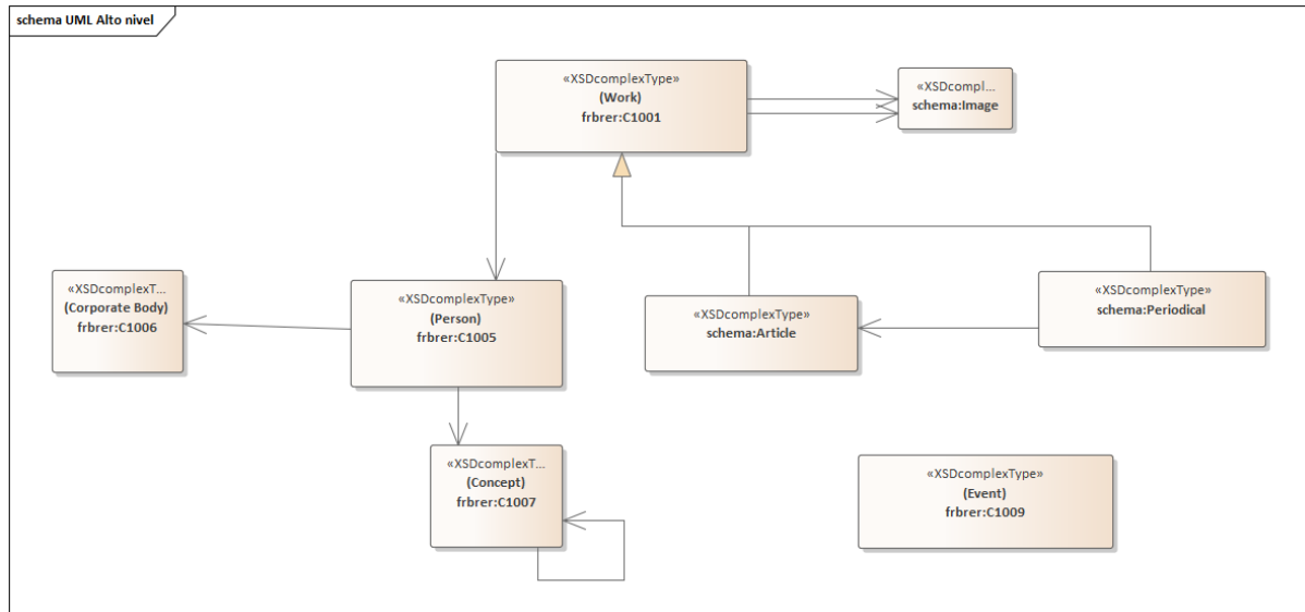
Figura 1 UML de alto nivel
